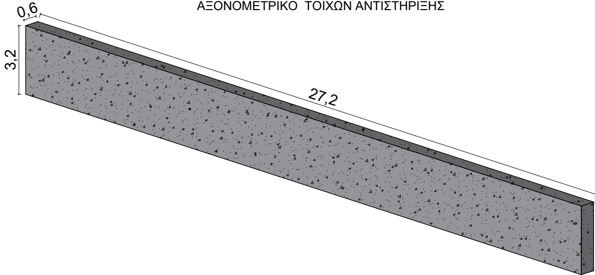
ΑΞΟΝΟΜΕΤΡΙΚΟ ΤΟΙΧΩΝ ΑΝΤΙΣΤΗΡΙΞΗΣ
