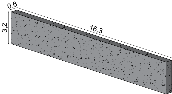
ΑΞΟΝΟΜΕΤΡΙΚΟ ΤΟΙΧΩΝ ΑΝΤΙΣΤΗΡΙΞΗΣ
